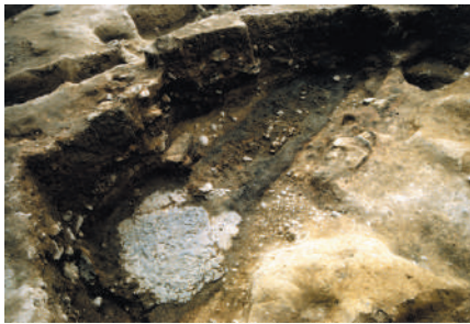
源内峠遺跡 製鉄炉 (滋賀県提供)
